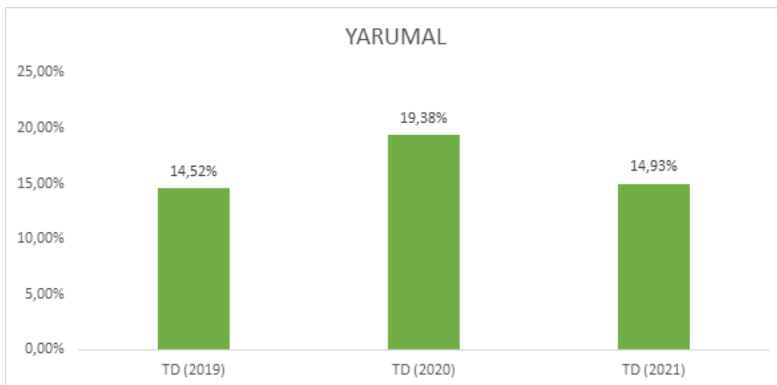
Gráfico 3. Evolución de la Tasa de Desempleo en Yarumal.
