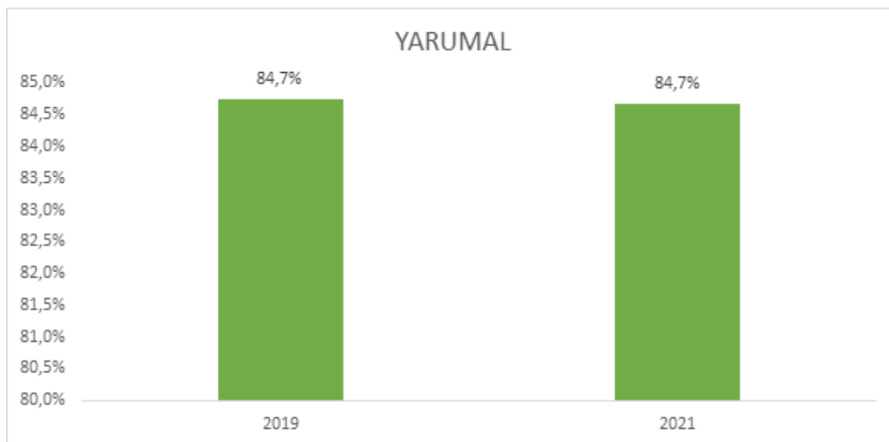
Gráfico 4. Evolución de la Tasa de Informalidad en Yarumal.
